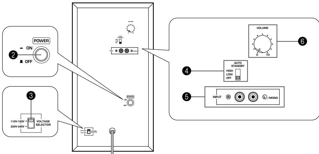
Achterpaneel
