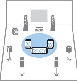
Monimittaus (5 kuuntelupaikkaa)
