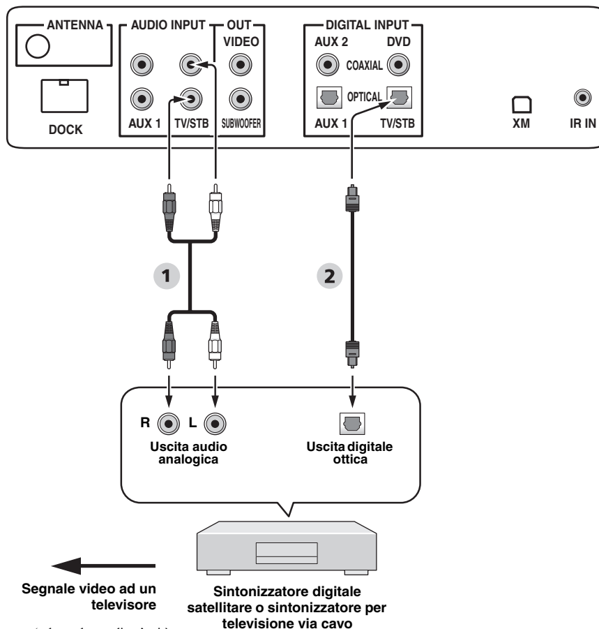
Pannello posteriore di quest'unità (Modelli per USA e Canada)
